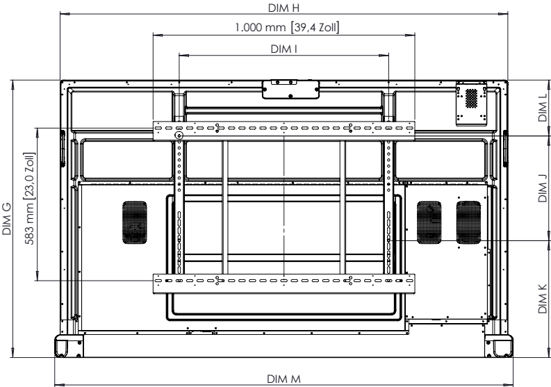
Rückansicht
